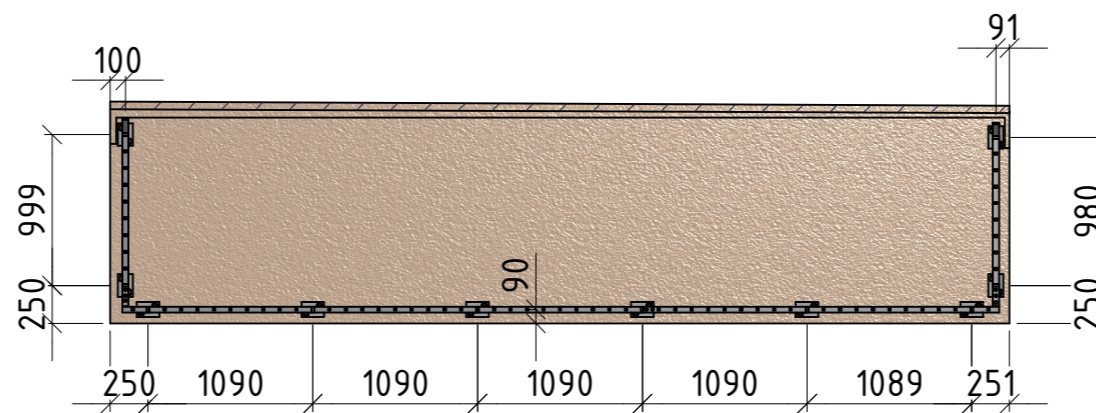
J-J ( 1 : 50 )
