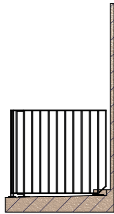
K-K ( 1 : 50 )
